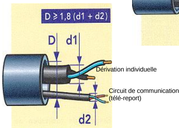
Diamètres des conduits pour les dérivation individuelles
